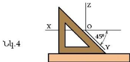
Շեղանկյուն դիմետրիա
